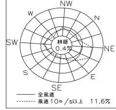
潮位図
