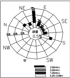
波向別波高出現頻度図
