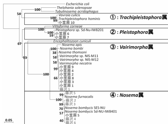
図2 小笠原（父島）と藤沢市で採集されたハスモンヨトウから得られた微胞子虫胞子のSSU rDNA 配列解析結果 a
