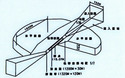
三宅島空港制限表面説明図
