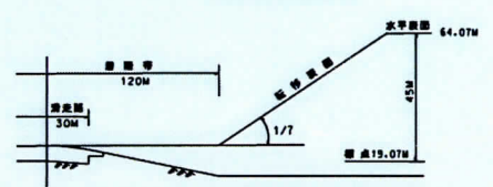
転移表面横断面図
