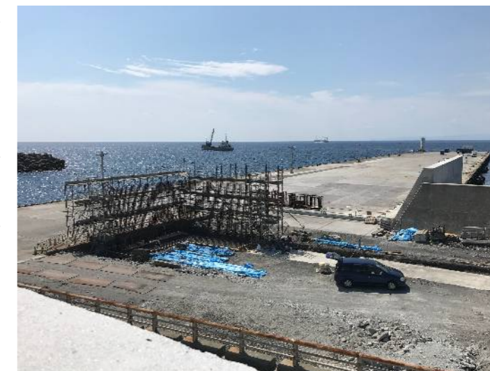
L型擁壁の建設状況
