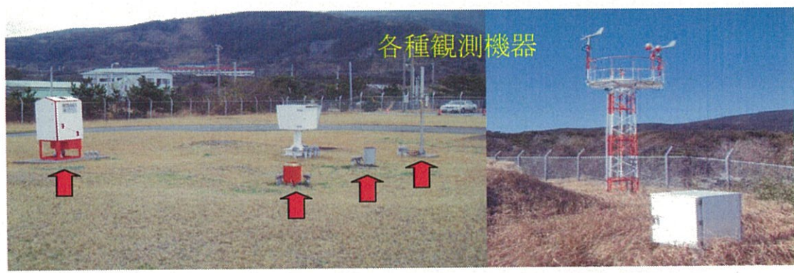
左から、シーロメーター※、雨量計、降雨強度計、温度計 ※ 雲の高さを測る機械です 風向・風速計 滑走路の両端にあります
