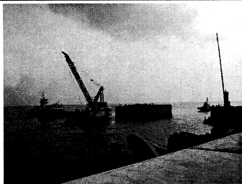
ケーソン据付状況（神湊漁港）
