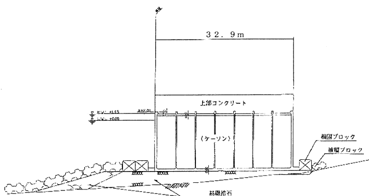
図- ケーソン断面図(神湊漁港)
