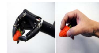
【高専が開発したロボットハンド】
